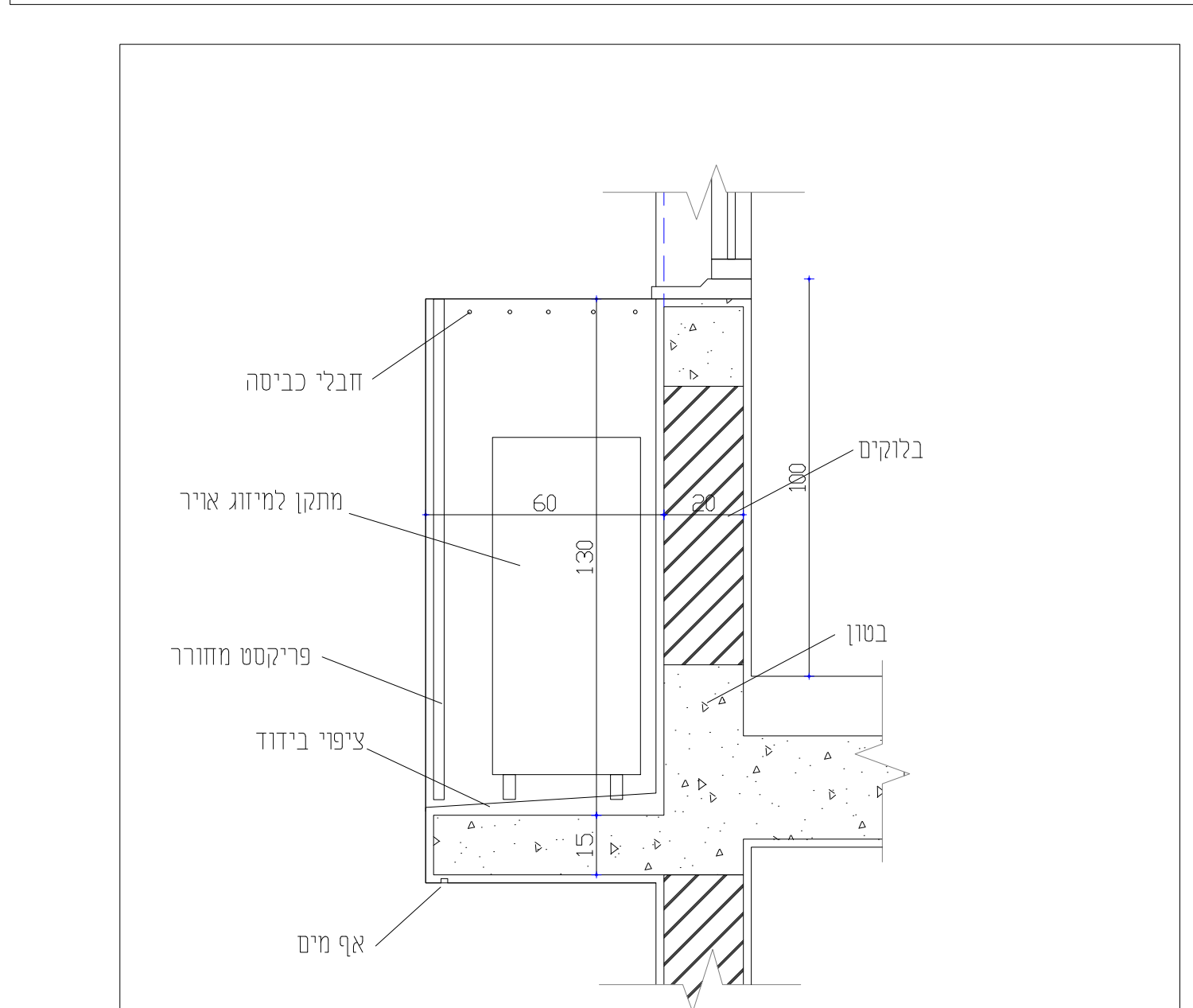
פרט מסתור כביסה ומזגנים קנה מידה 1:20
